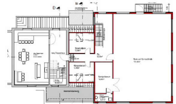
GRUNDRISS 1.OBERGESCHOSS
